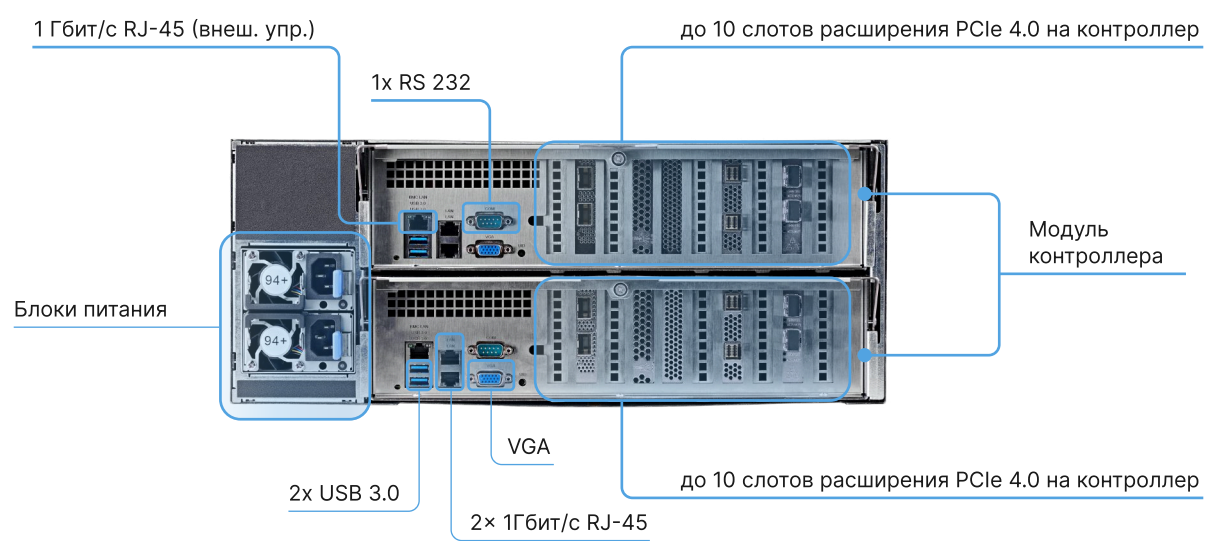
Архитектура платформы. Расположение портов.
