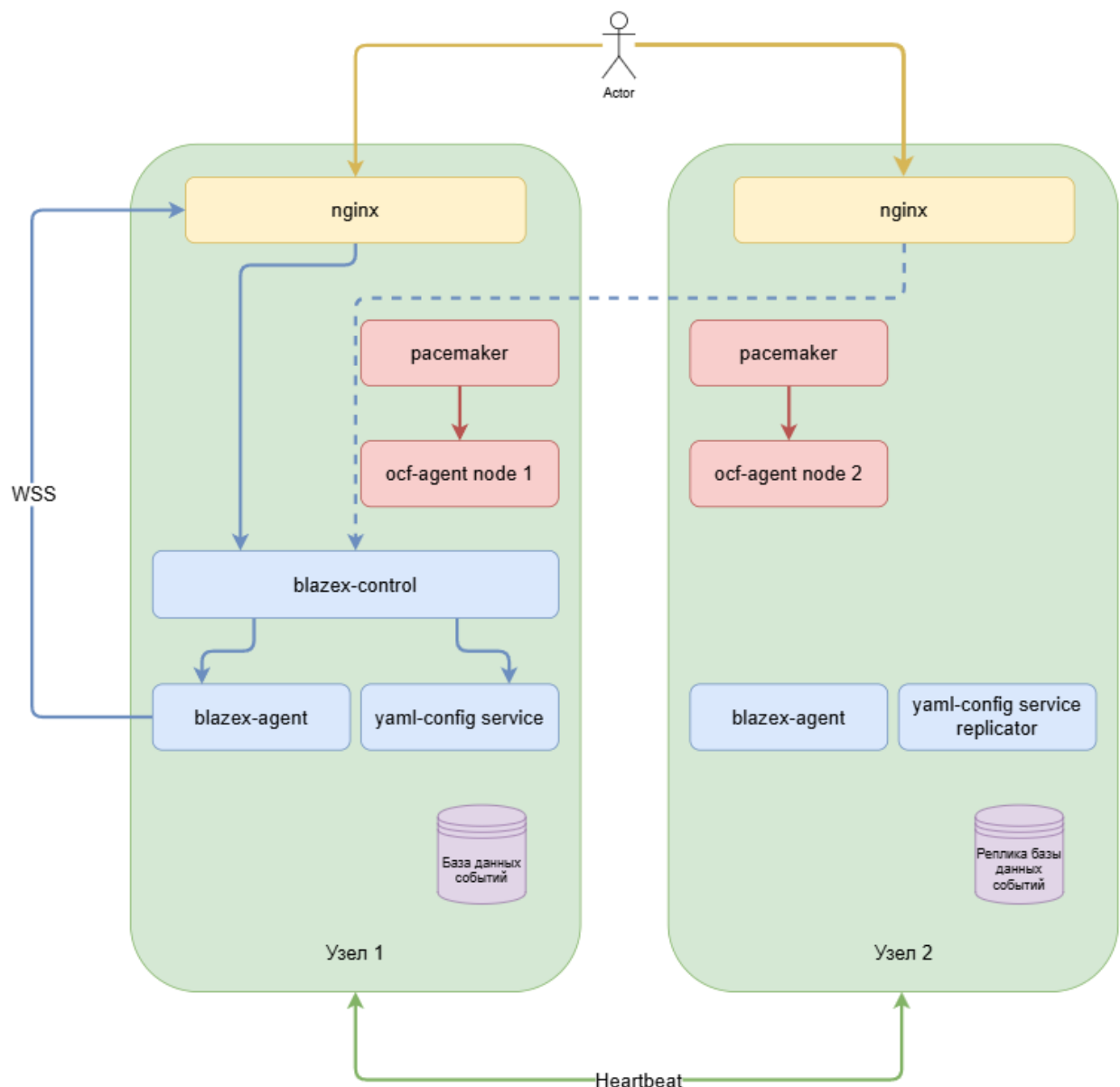
Рисунок 1 - схема архитектуры управляющего ПО BlazeX
